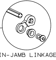
IN-JAMB LINKAGE
